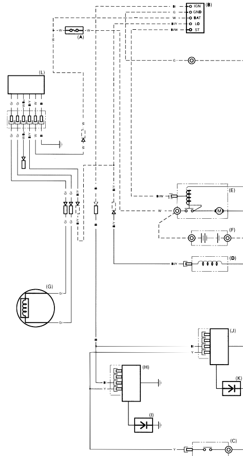
Type à bobine de charge 17 A et sans boîte de commande
