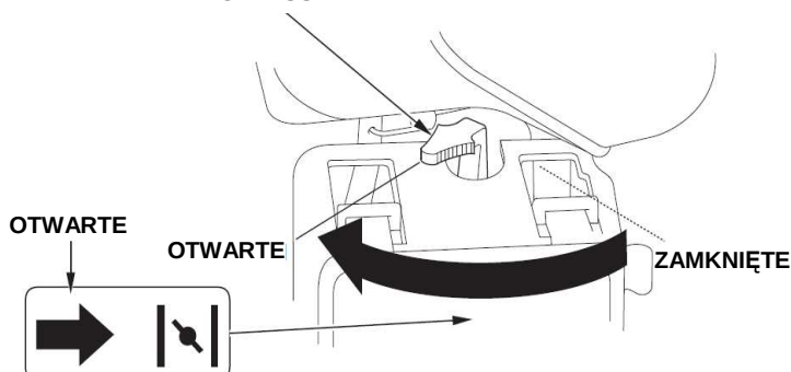
DŹWIGNIA SSANIA
